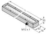
Линейная подсветка Тип: LEDBLA435SSD6-XQ Идент. №: 3013522
